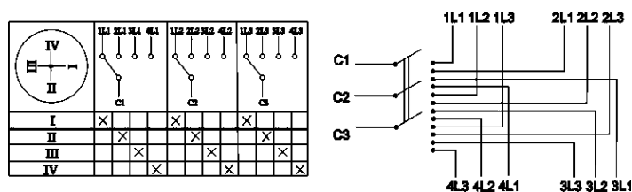
Пакетный переключатель ПП 3-полюсный на 4 направления
