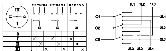
Пакетный переключатель ПП 3-полюсный на 3 направления
