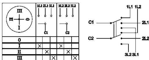
Пакетный переключатель ПП 2-полюсный на 3 направления
