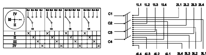
Пакетный переключатель ПП 4-полюсный на 4 направления
