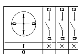
Пакетный выключатель ПВ 3-полюсный
