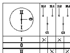
Пакетный переключатель ПП 2-полюсный на 2 направления
