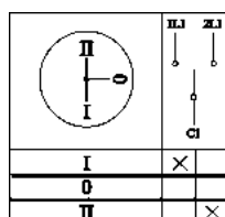
Пакетный переключатель ПП 1-полюсный на 2 направления
