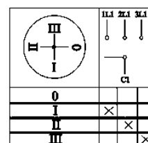
Пакетный переключатель ПП 1-полюсный на 3 направления
