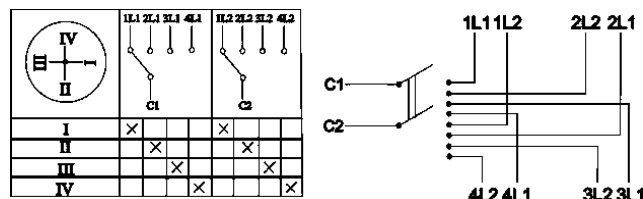
Пакетный переключатель ПП 2-полюсный на 4 направления
