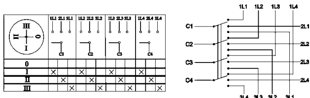
Пакетный переключатель ПП 4-полюсный на 3 направления
