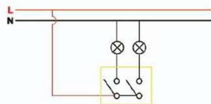
Схема цепи / Wiring Diagram
