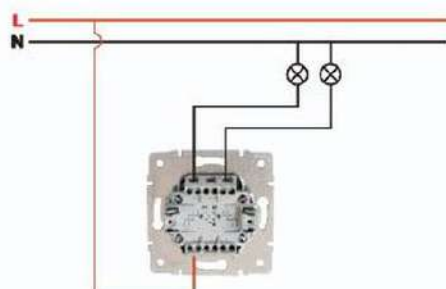
Схема подсоединения / Connection Diagram
