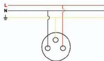
Схема цепи / Wiring Diagram
